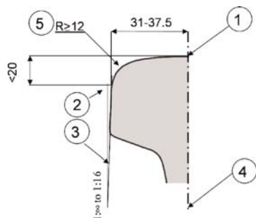
Profil hlavy koľajnice
